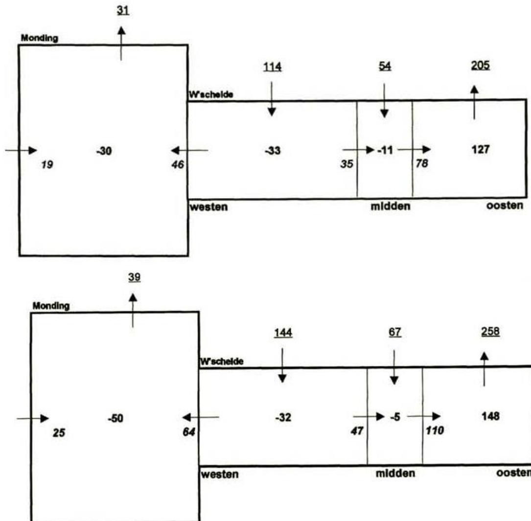
Figuur 3.28 Sedimentbalans [miljoen m³] over de periode 1999-2030 zonder ZSS (bovenste paneel) en over de periode 1999-2038 met ZSS van 0,6 m/eeuw (onderste paneel). (figuren afkomstig uit Jeuken et al., 2002)
